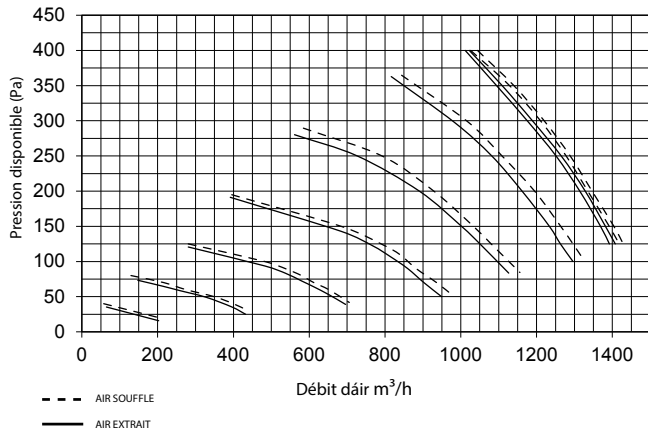
Courbe caractéristique des ventilateurs d'air extrait et d'air soufflé LTR-7 avec filtres M5/M5 filters
